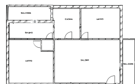
Planimetria appartamento di 70 mq
